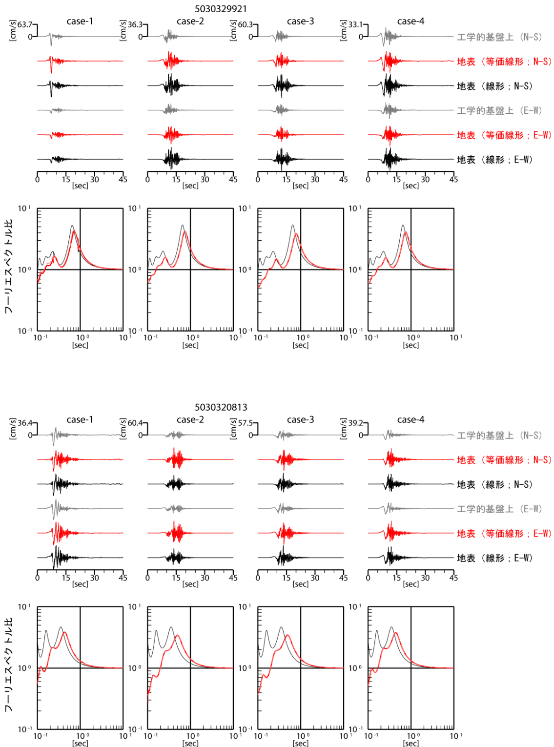
図 33-2 2005 年福岡県西方沖の地震に関する応答計算結果による、埋め立て地の軟弱地盤における速度波形および「地表／工学的基盤上面」のフリーエスペクトル比 地点は海の中道 (5030329921 ; 上段) と百道浜 (5030320813 ; 下段)
