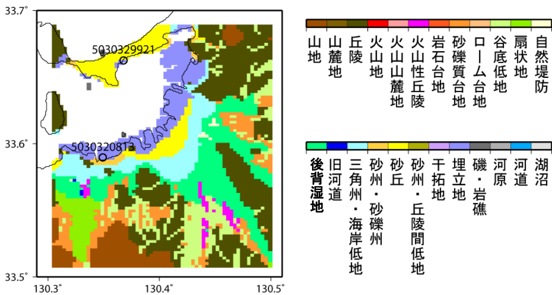
図 32-2 軟弱地盤における波形・スペクトル比の比較を行う地点（○） 背景は若松・他（2007）による地形区分
