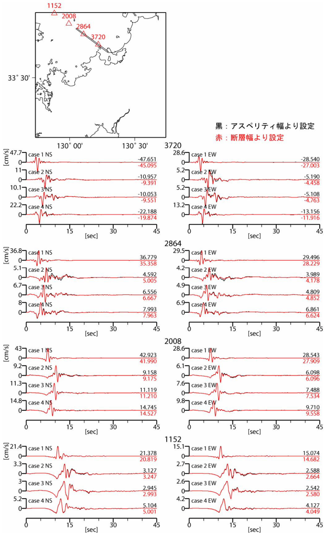
図 21-2 ライズタイムの違いによる計算波形の比較（破壊進行の反対方向の観測点） （工学的基盤における速度波形）
