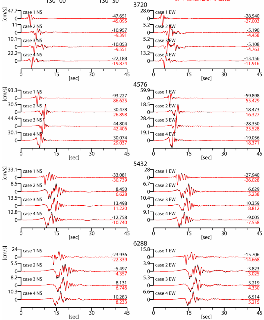
図 21-1 ライズタイムの違いによる計算波形の比較（破壊の進行方向の観測点） （工学的基盤における速度波形）
