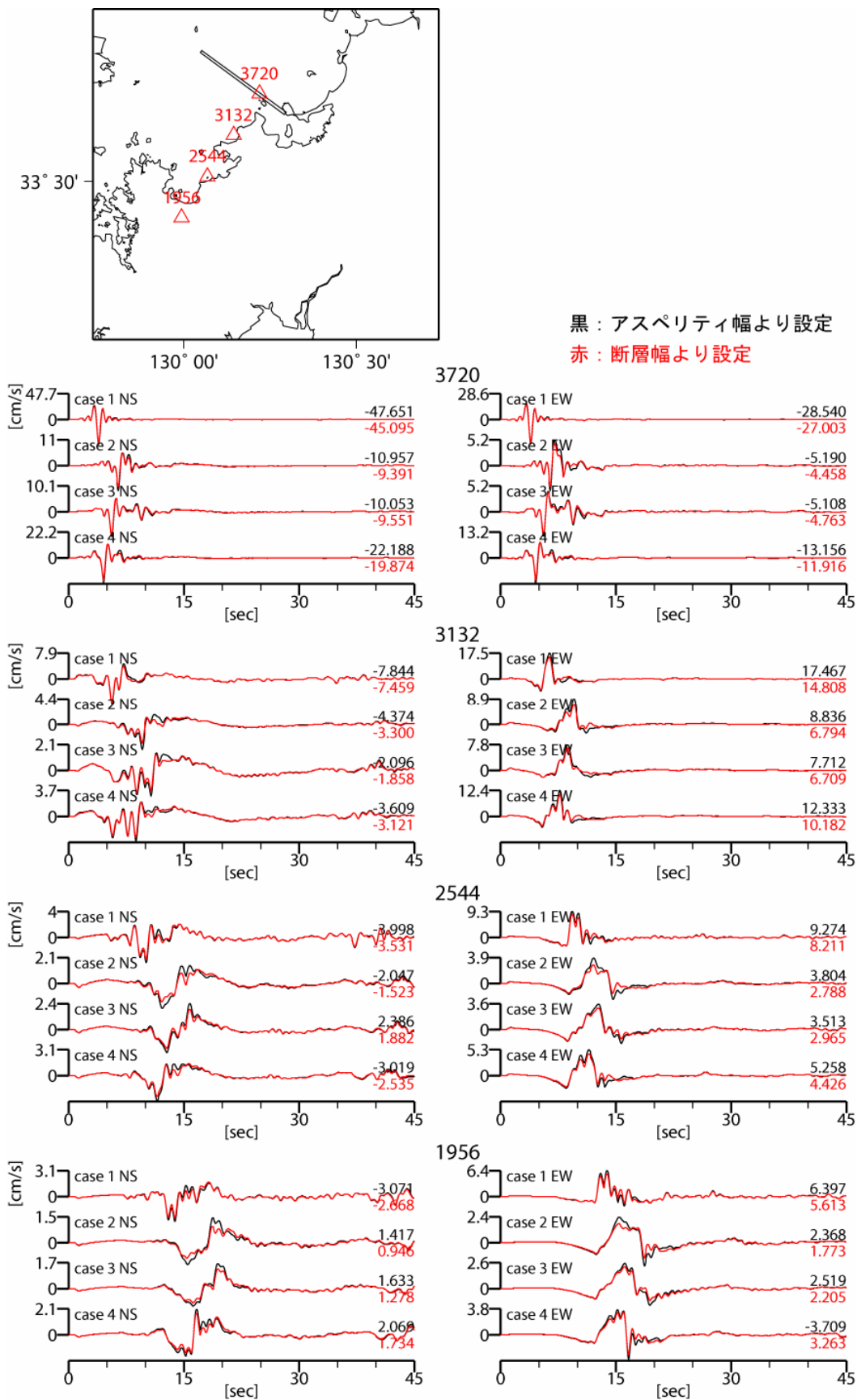
図 21-3 ライズタイムの違いによる計算波形の比較（断層に直交する方向の観測点） （工学的基盤における速度波形）
