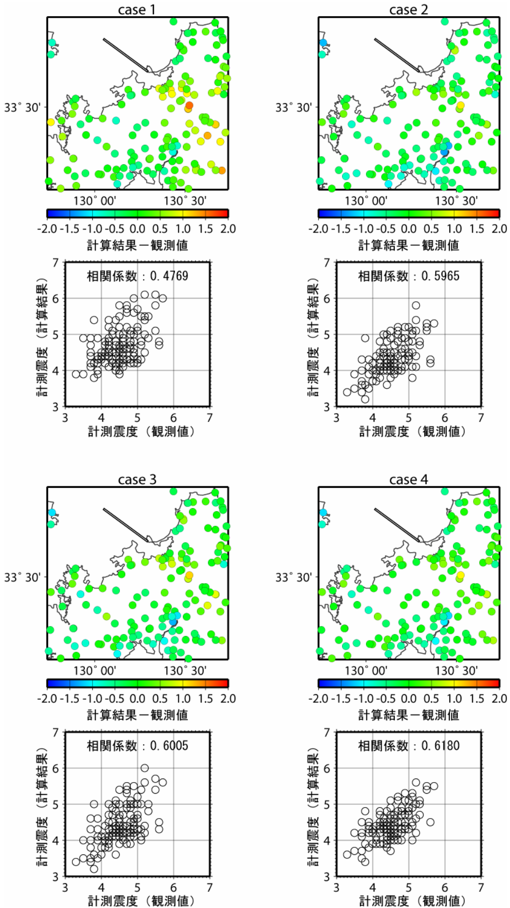
図 16 ハイブリッド合成法による計算結果と観測記録の比較（地表の計測震度）
