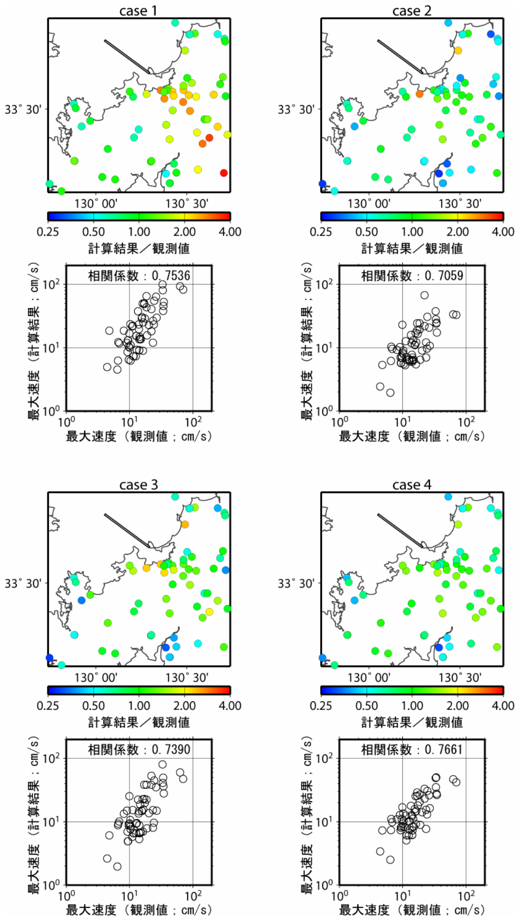
図 15 ハイブリッド合成法による計算結果と観測記録の比較（地表の最大速度）
