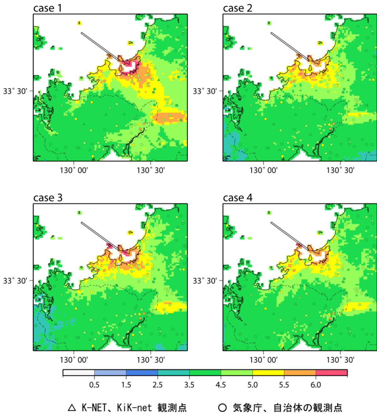
図 14 ハイブリッド合成法による計測震度分布
