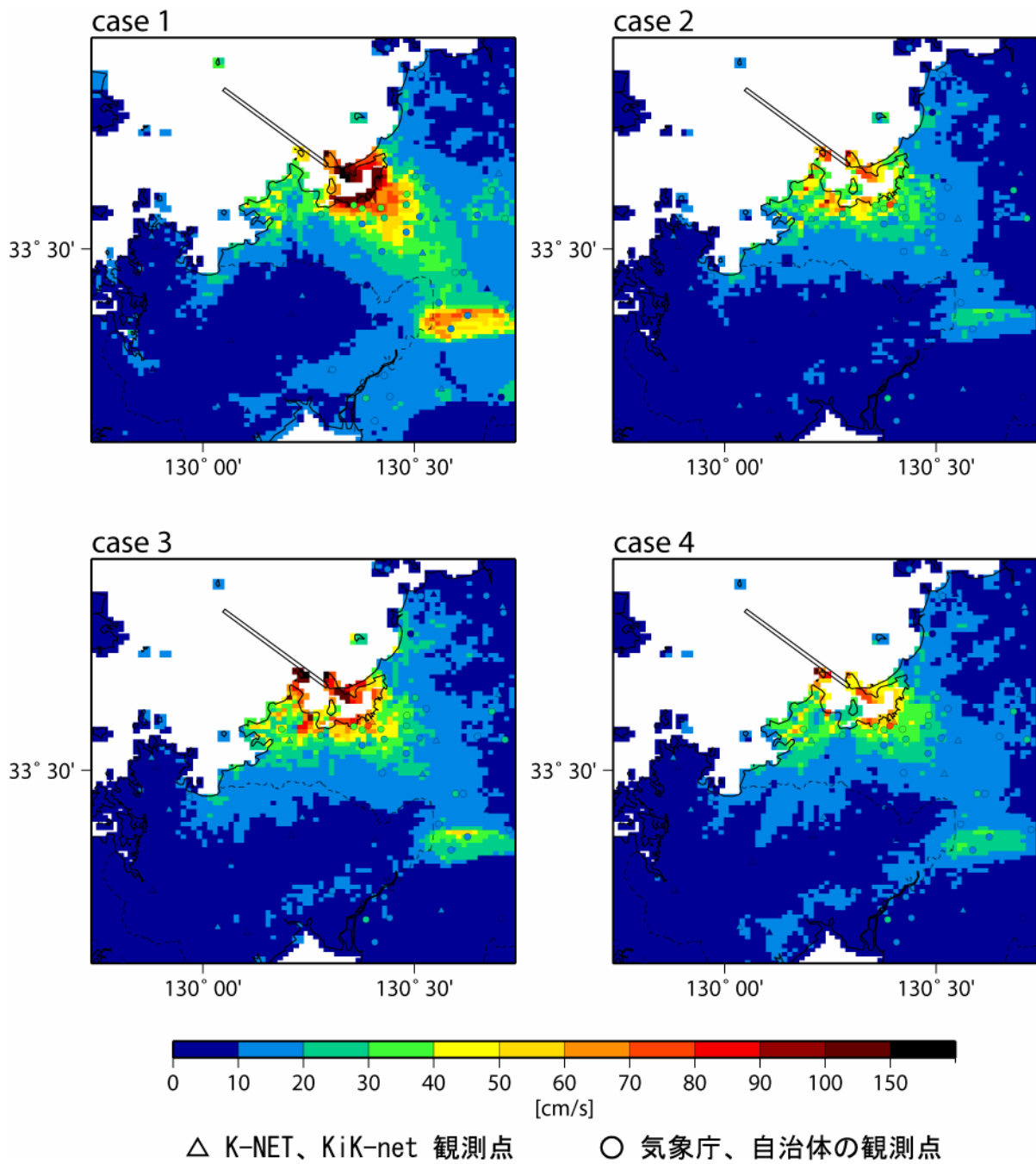
図 13 ハイブリッド合成法による地表における最大速度分布
