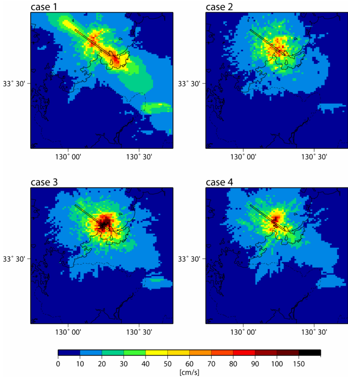
図 12 ハイブリッド合成法による工学的基盤における最大速度分布
