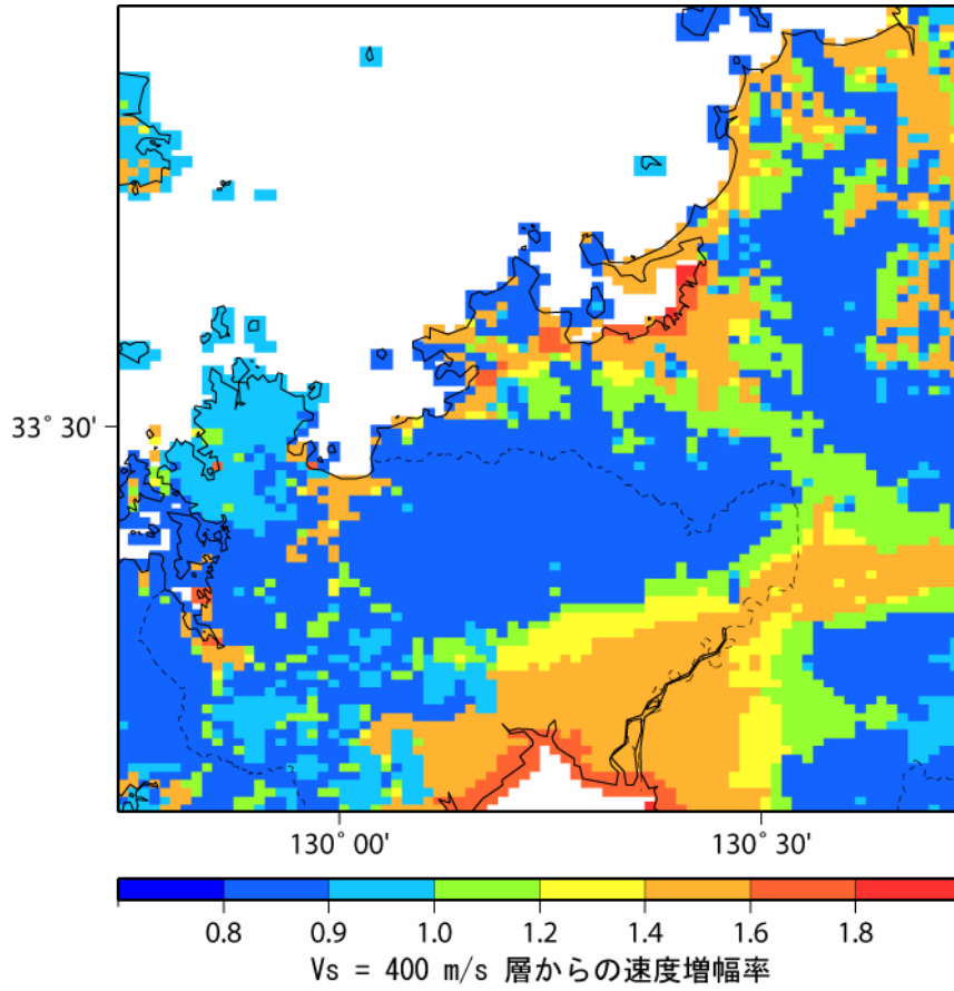
図 11 浅い地盤構造（藤本・翠川（2003）の手法による最大速度の増幅率）
