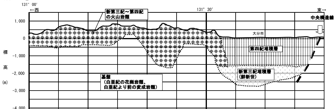
図4 堆積層の模式断面図
