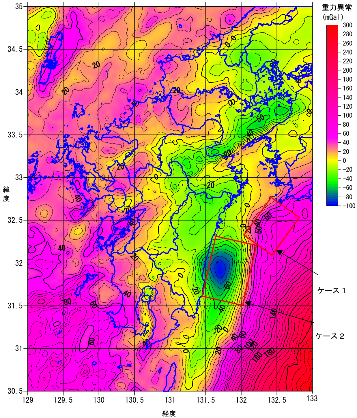
図 1 4 想定した震源断層とブーゲー異常図 (産業技術総合研究所, 2004 に加筆)
