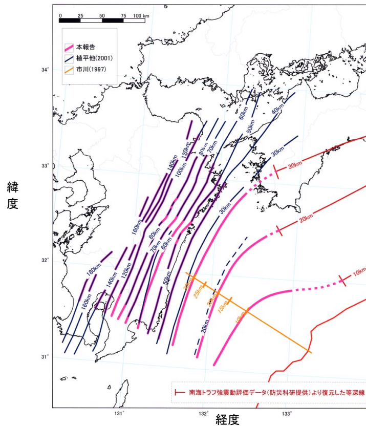
図 1 2 微小地震の震源分布にもとづくプレート境界面の推定等深線図 (地震調査委員会, 2004)
