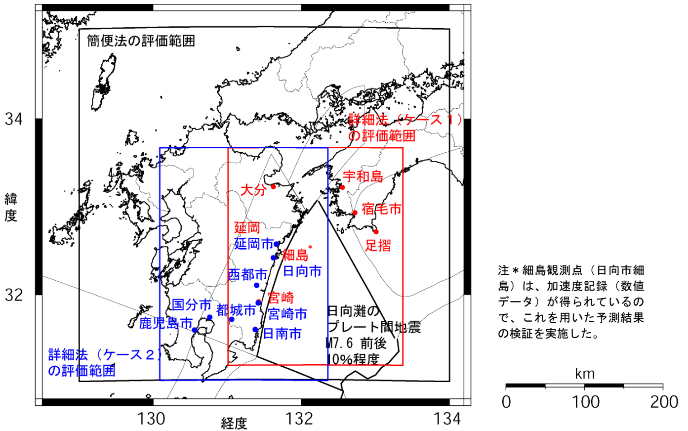
図 1 1 「長期評価」による日向灘の地震の震源域の範囲・規模・地震のタイプ・30 年地震発生確率 (2005 年 1 月 1 日起点)、強震動評価領域、及び計算波形を示す代表地点
