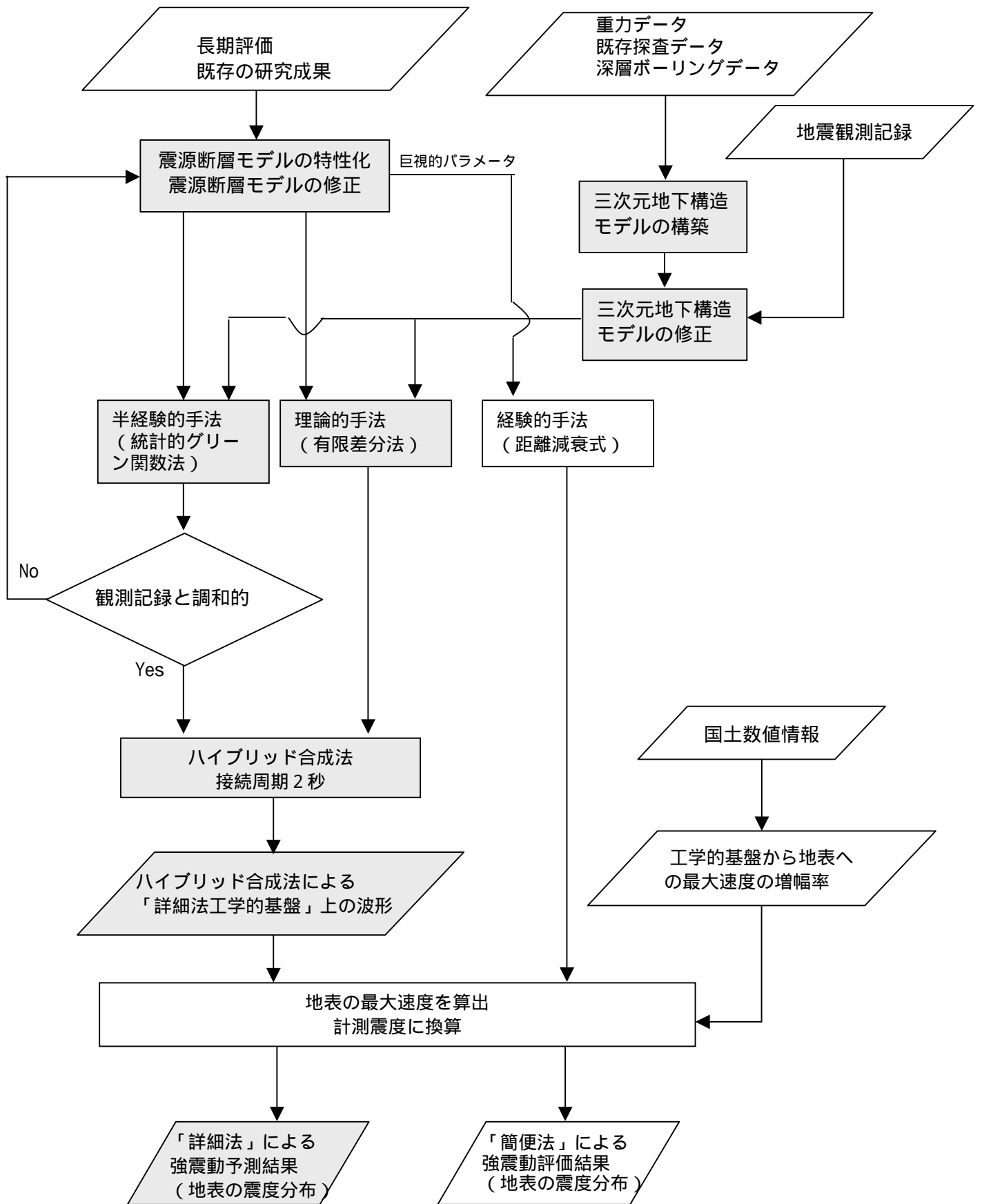
図10 強震動評価の流れ（網掛けは「詳細法」の処理）
