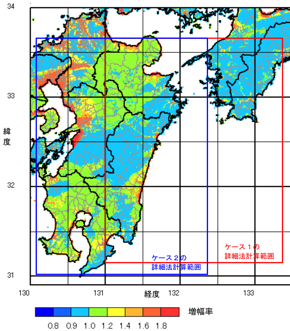
図5 「浅い地盤構造」(詳細法工学的基盤( V_s=500\text{m/s} )から地表まで)における最大速度の増幅率
