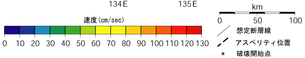
図18-1 「詳細法」による強震動予測結果：「詳細法工学的基盤」上の最大速度分布 (モデル1：ケース1-1、1-2、1-3)
