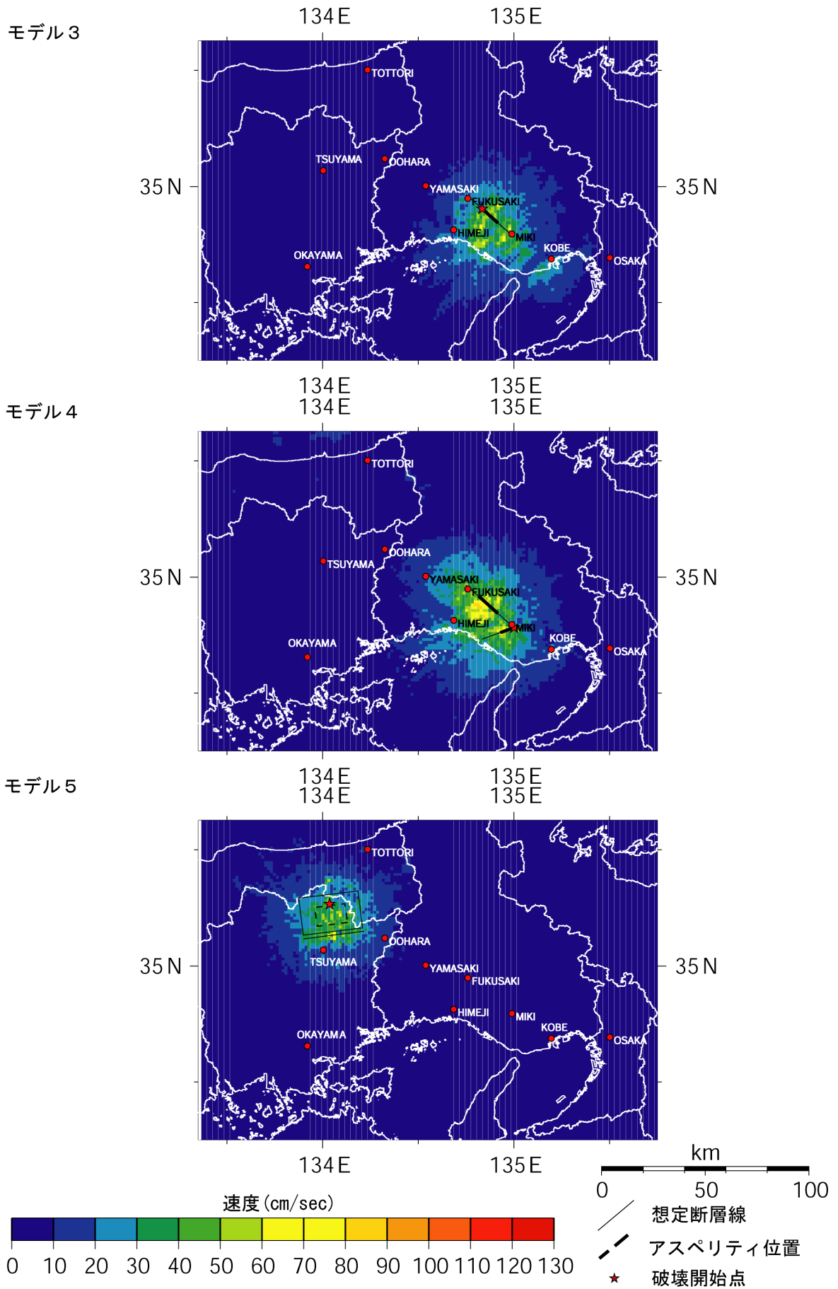
図18-3 「詳細法」による強震動予測結果：「詳細法工学的基盤」上の最大速度分布 (モデル3、モデル4、モデル5)
