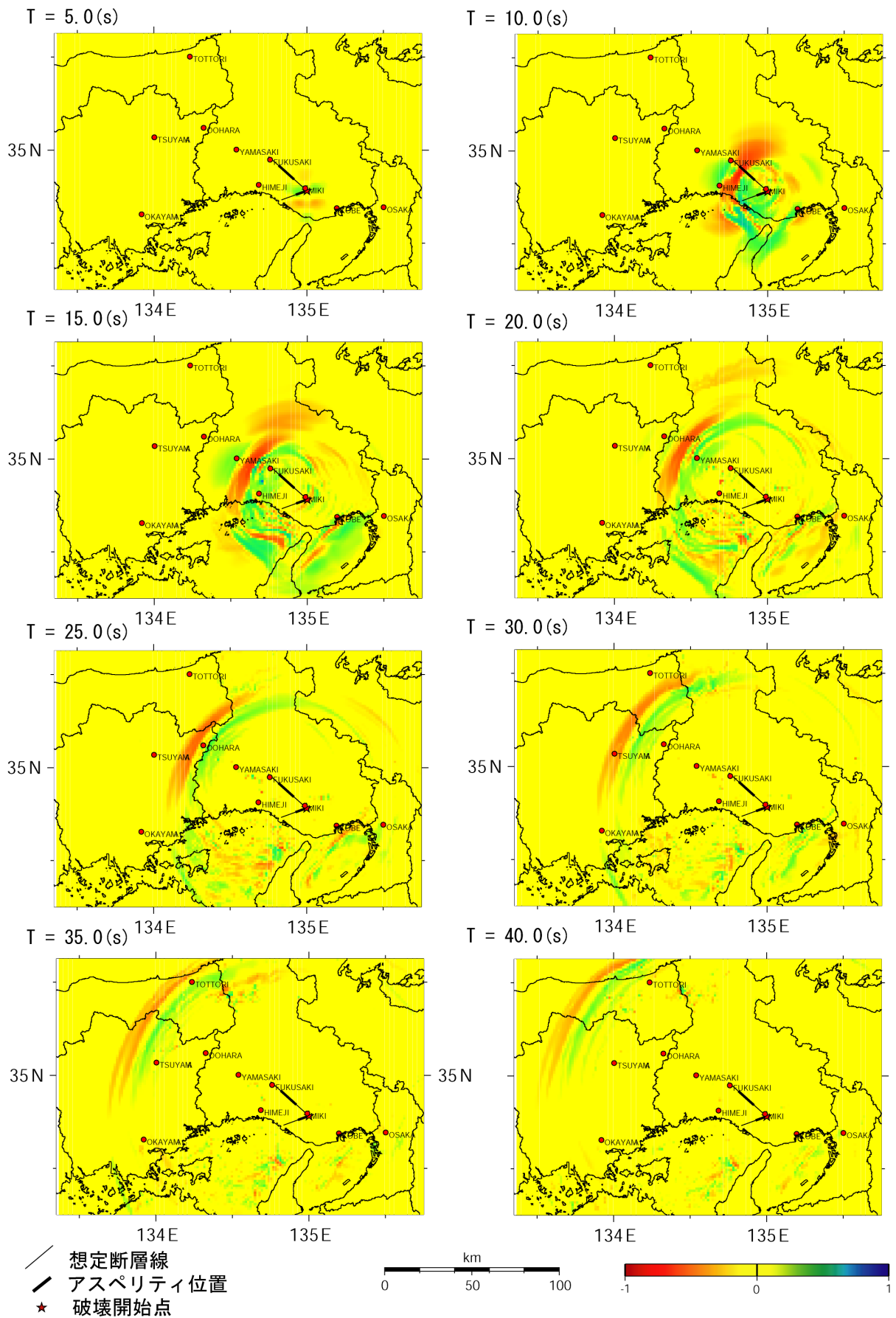
図 15-5 有限差分法による計算結果例（モデル4、「詳細法工学的基盤」 ( V_s=550\text{m/s} 、 V_s=590\text{m/s} ) 上の速度振幅のスナップショット、NS 成分)
