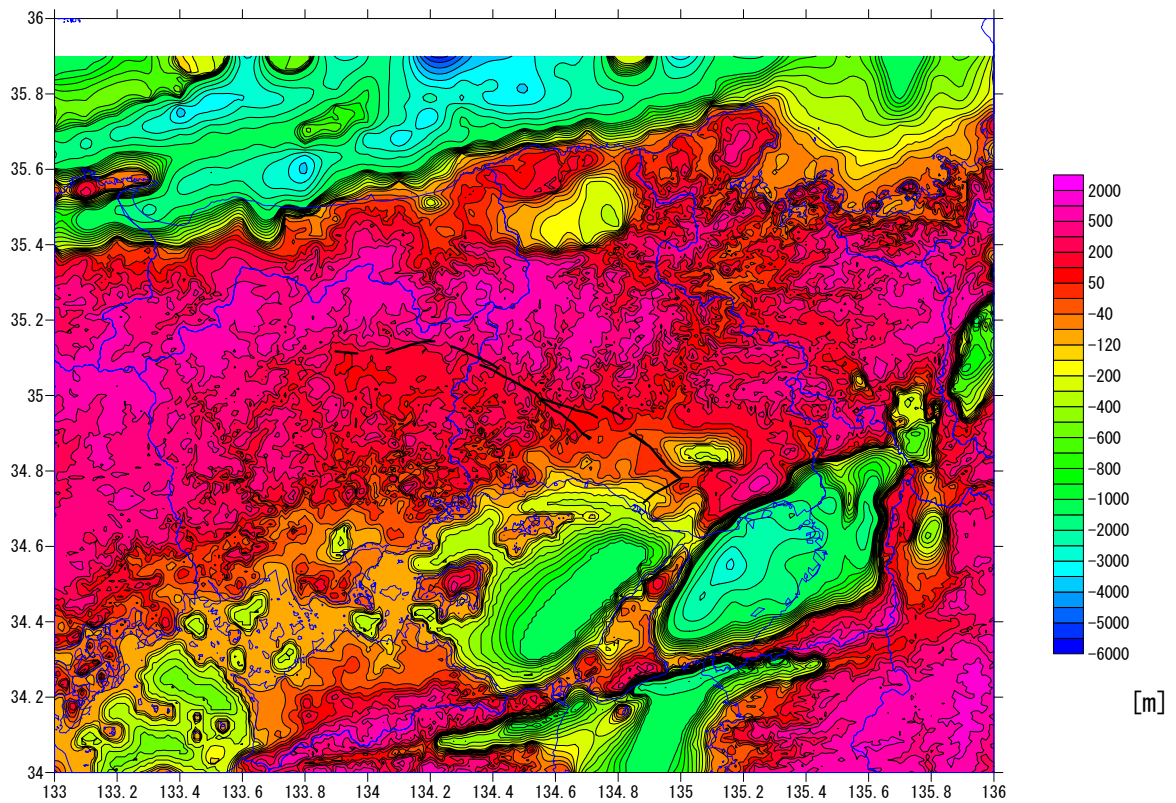
図 1 3 - 3 想定した震源断層の周辺地域における「深い地盤構造」の速度層構造 (速度層上面標高コンター、上 : V_p=3.3\text{km/s} ( V_s=1.3\text{km/s} )、下 : V_p=3.8\text{km/s} ( V_s=1.6\text{km/s} ))
