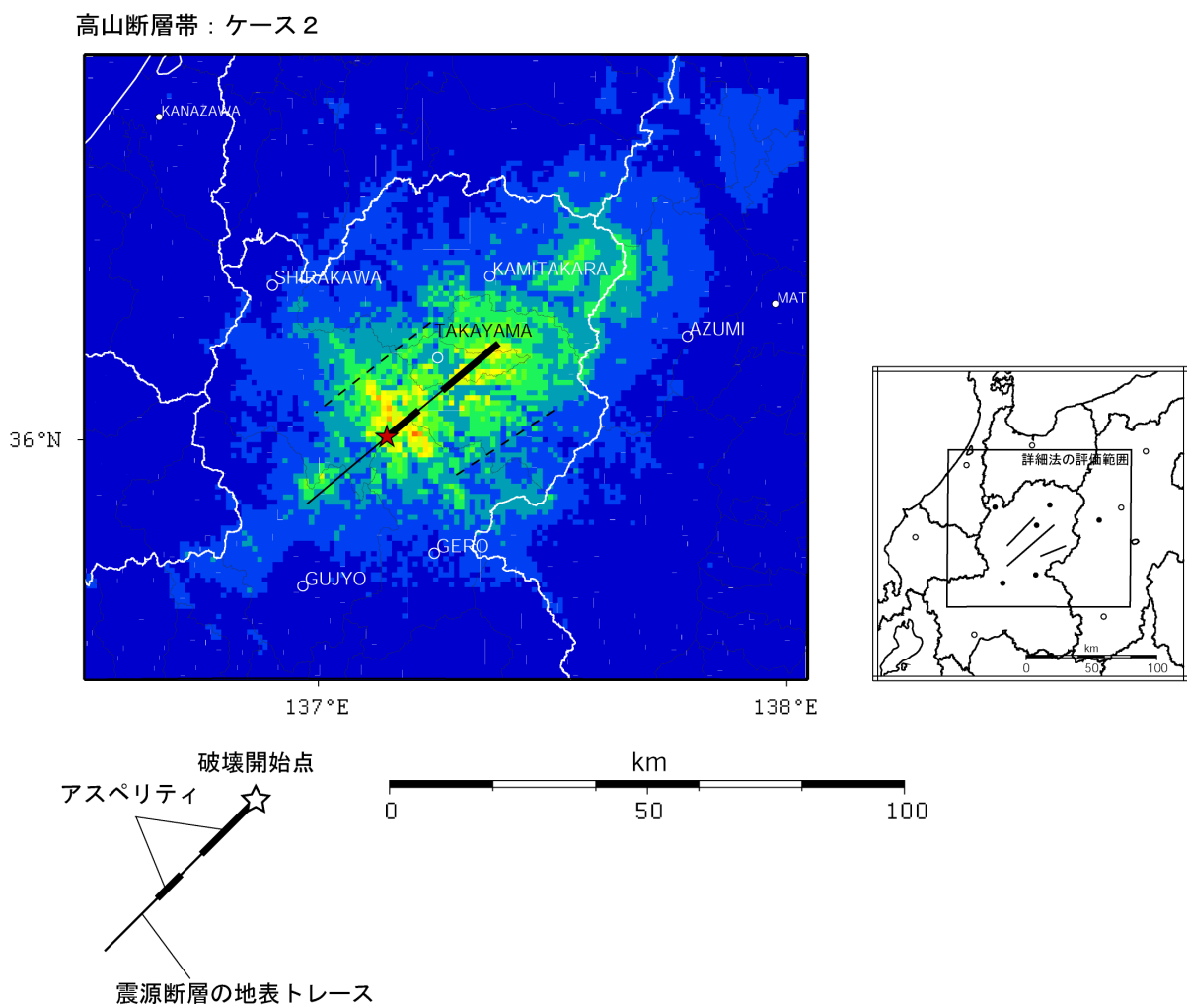
図 18-1 「詳細法」による強震動予測結果：「詳細法工学的基盤」上の最大速度分布 (高山断層帯：ケース 1, 2)
