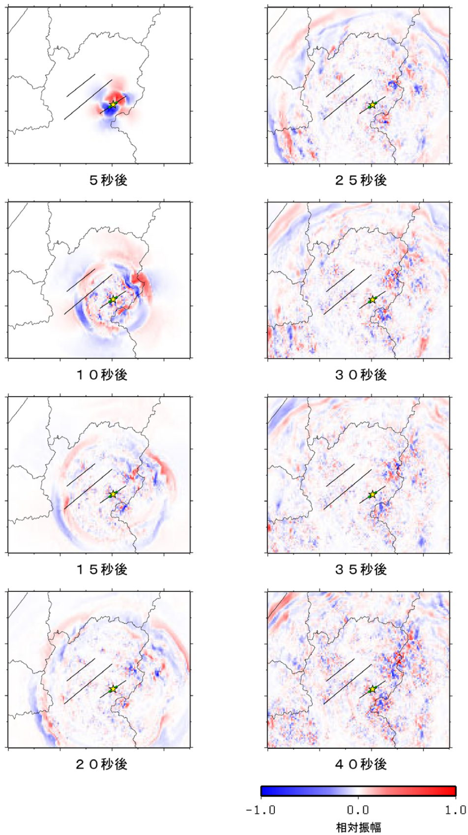
図 1 5 - 5 有限差分法による計算結果例（猪之鼻断層帯、「詳細法工学的基盤」( V_s=750\text{m/s} ) 上の速度振幅のスナップショット、NS 成分)
