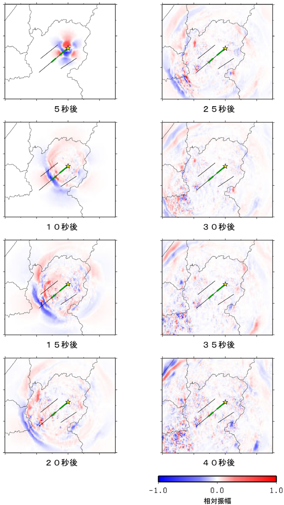
図 1 5 - 1 有限差分法による計算結果例（高山断層帯、ケース 1、「詳細法工学的基盤」 ( V_s=750\text{m/s} ) 上の速度振幅のスナップショット、NS 成分)
