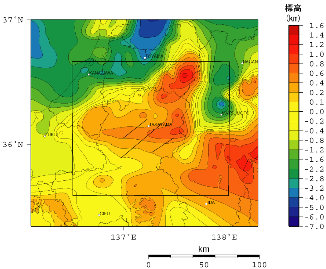
図14-2 想定した震源断層の周辺地域における「深い地盤構造」の速度層構造 (速度層上面標高コンター、上 : V_p=4.7 km/s ( V_s=2.2 km/s)、下 : V_p=5.9 km/s ( V_s=3.46 km/s))
