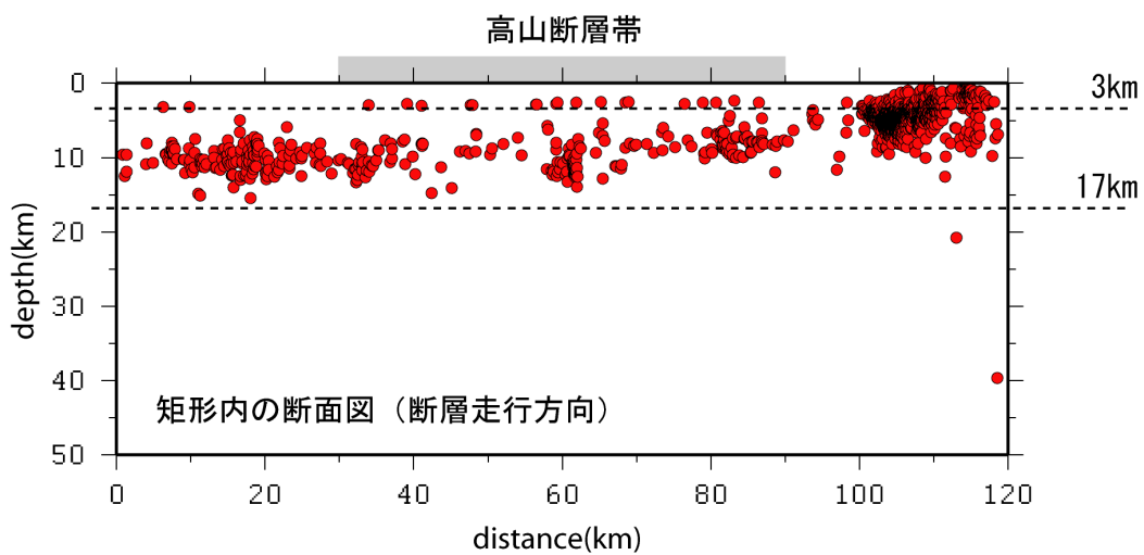
図10 高山・大原断層帯付近の微小地震分布 (1996.1~2003.10、気象庁の震源データによる)
