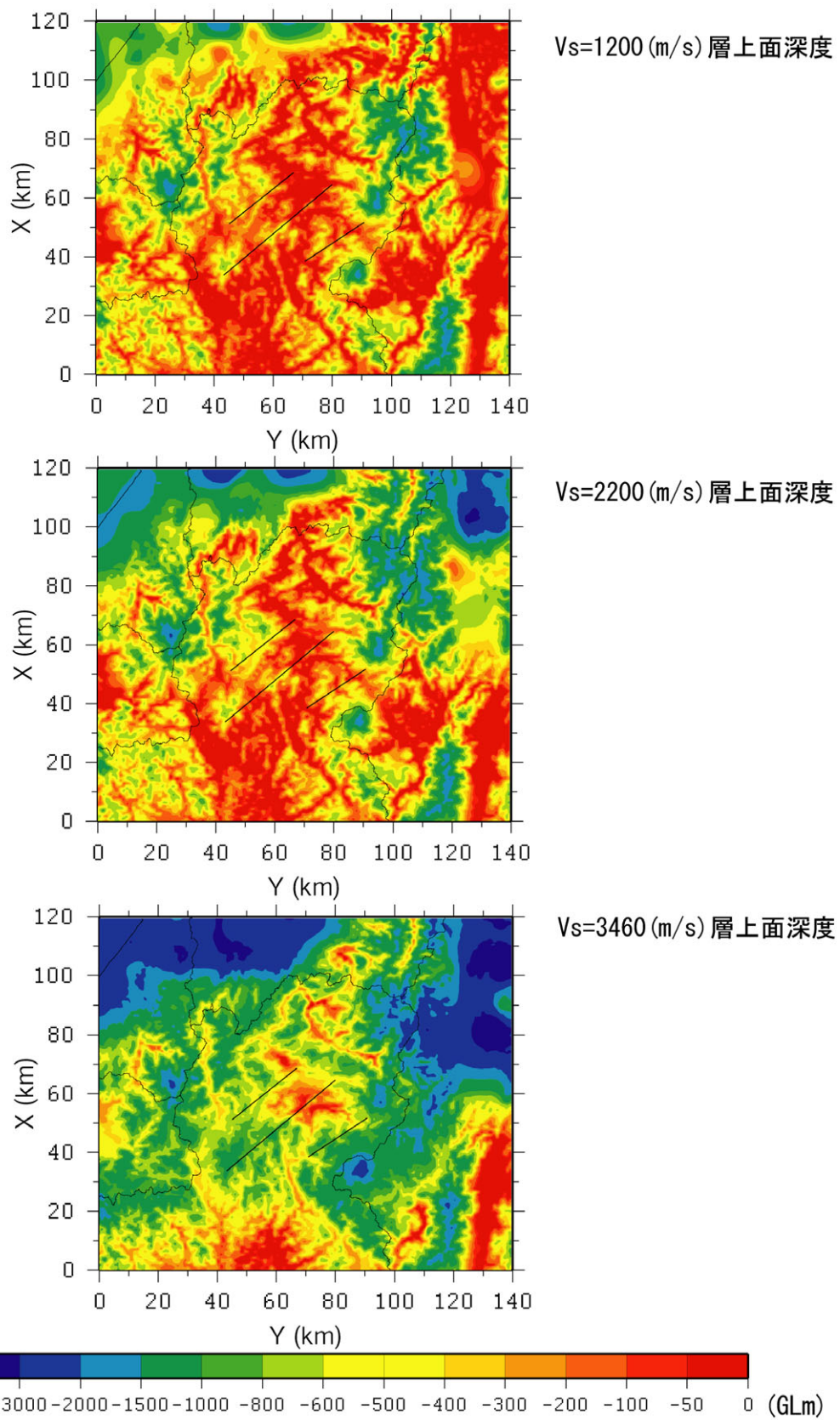
図3 「深い地盤構造」に用いた3次元地下構造モデル(各速度層上面の深さ分布[GLm])
