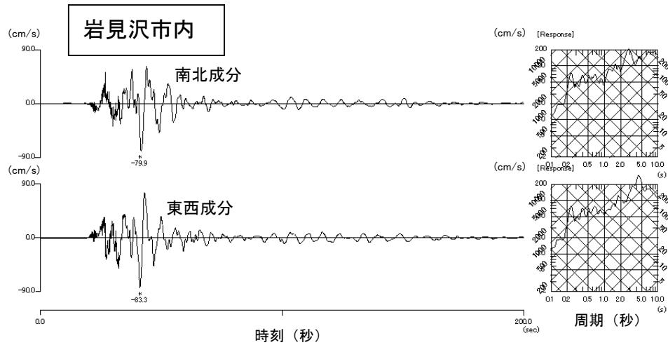
図 2 3 - 1 工学的基盤の速度波形と擬似速度応答スペクトル
