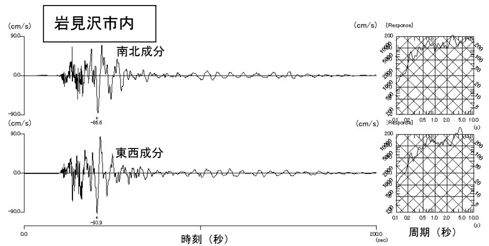
図 2 3 - 2 一次元地震応答計算による地表の速度波形と擬似速度応答スペクトル
