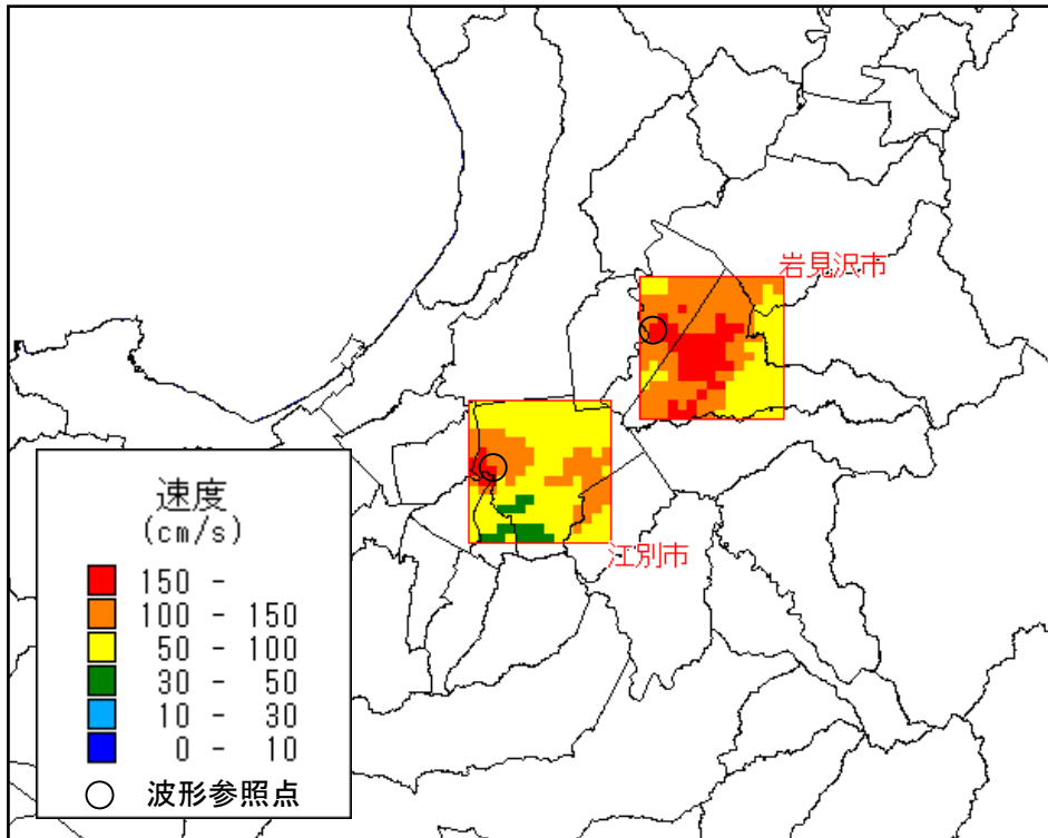
図 2 1 - 1 微地形分類による増幅率により求めた地表の最大速度分布
