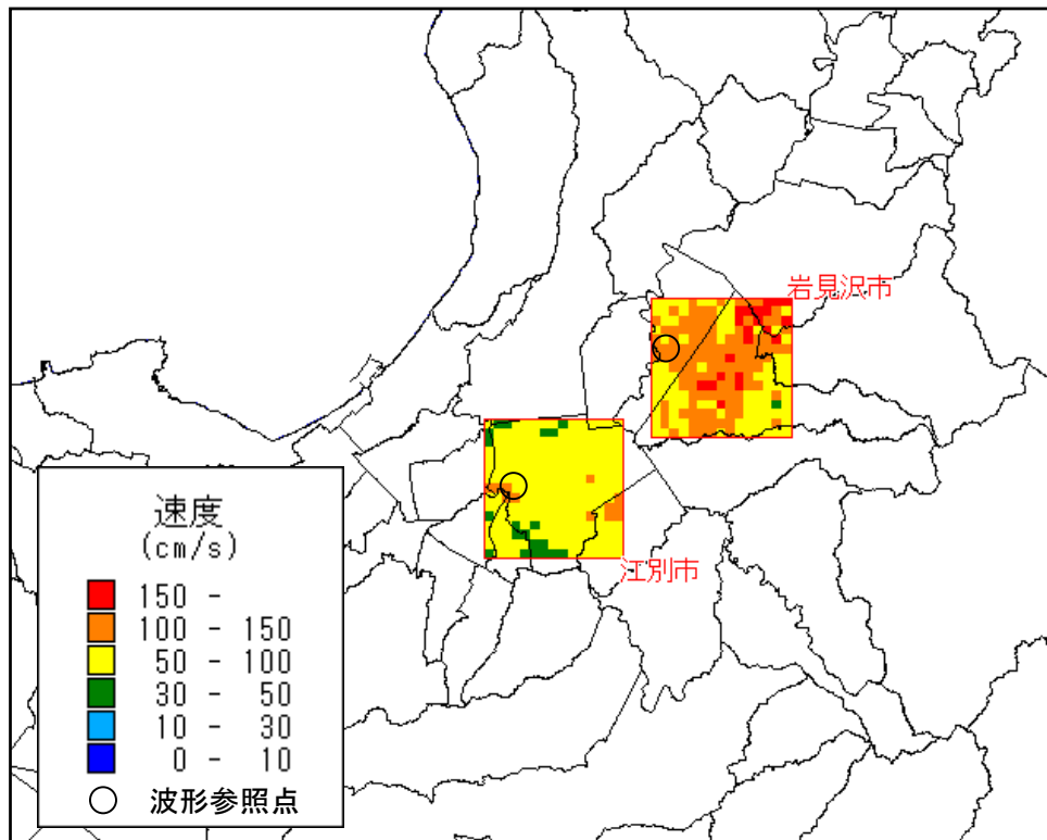
図 2 1 - 2 一次元地震応答計算による地表の最大速度分布
