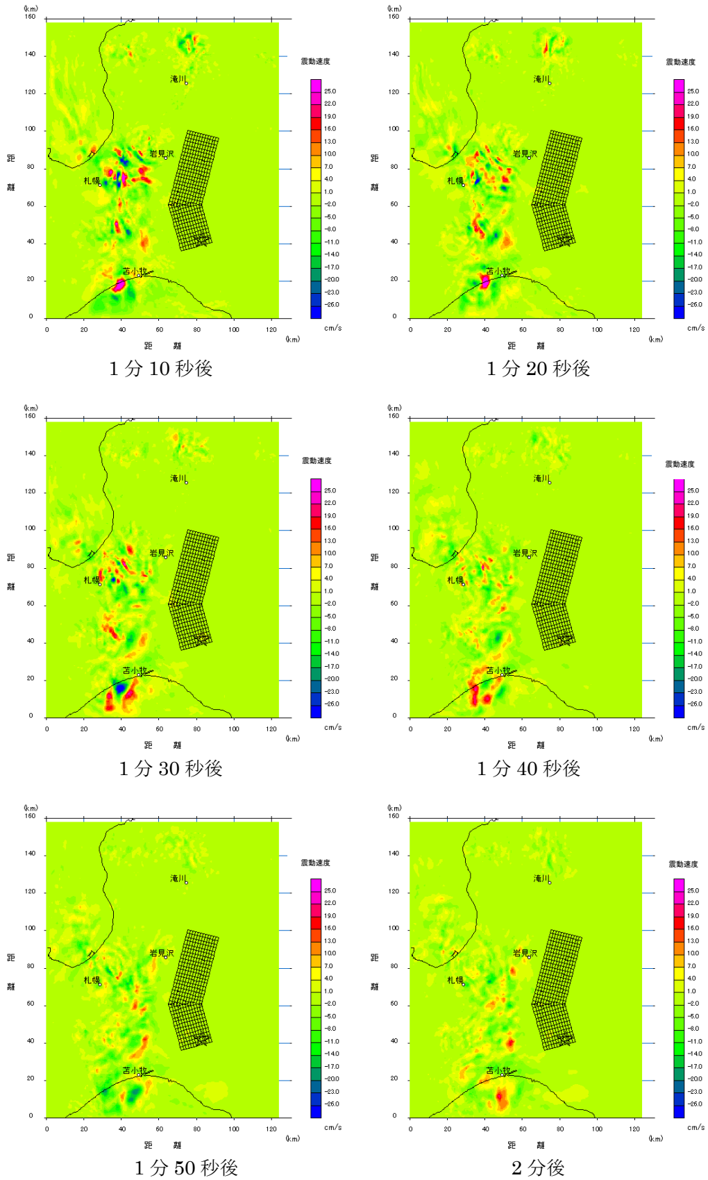
図 17-2 破壊開始1分10秒後から2分後までの工学的基盤面における速度振幅のスナップショット（ケース2, NS成分）
