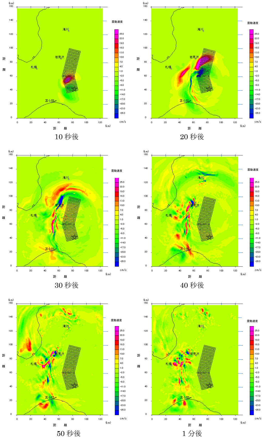
図 17-1 破壊開始10秒後から1分後までの工学的基盤面における速度振幅のスナップショット（ケース2, NS成分）
