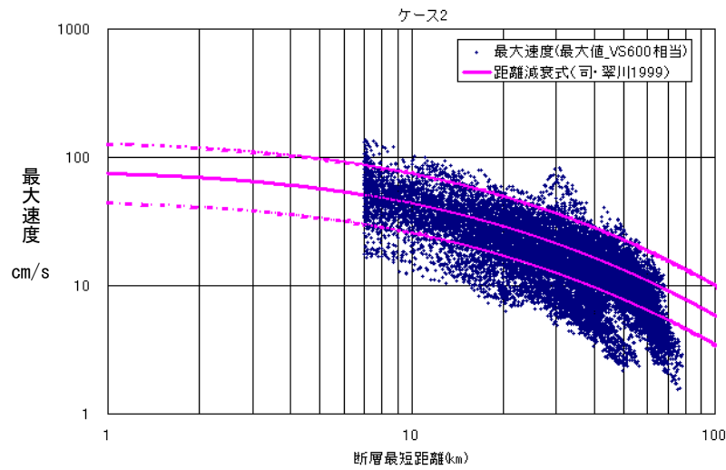
図 16-5 「詳細法工学的基盤」( V_s=480\text{m/s} )における最大速度値を V_s=600\text{m/s} 相当に補正した値と 司・翠川(1999)の距離減衰式との比較(ケース1~4)
