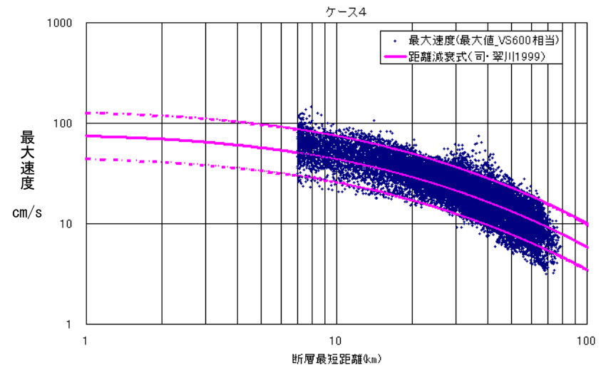
図 16-5 「詳細法工学的基盤」( V_s=480\text{m/s} )における最大速度値を V_s=600\text{m/s} 相当に補正した値と 司・翠川(1999)の距離減衰式との比較(ケース1~4)
