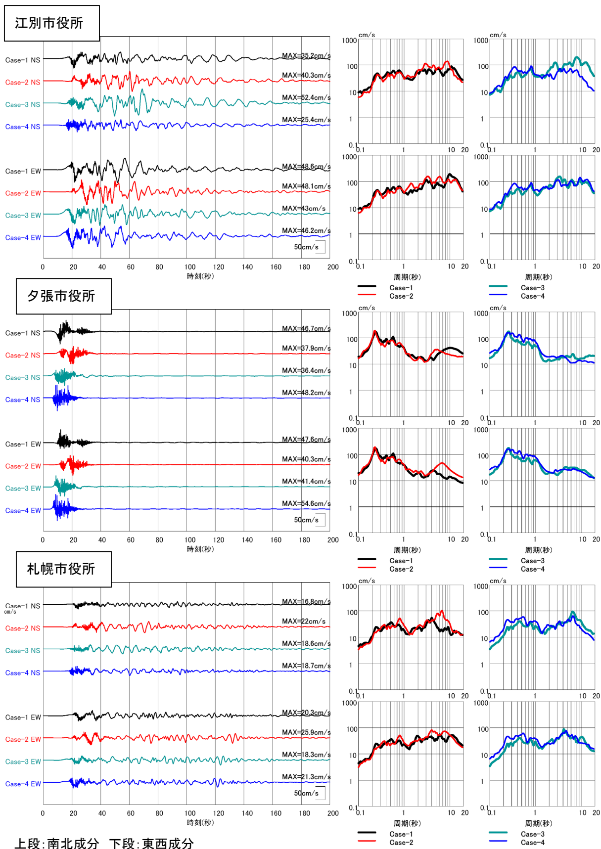
図 1 4 - 2 「詳細法工学的基盤」における計算波形と減衰 5 % 擬似 速度応答スペクトル (江別市役所・夕張市役所・札幌市役所)
