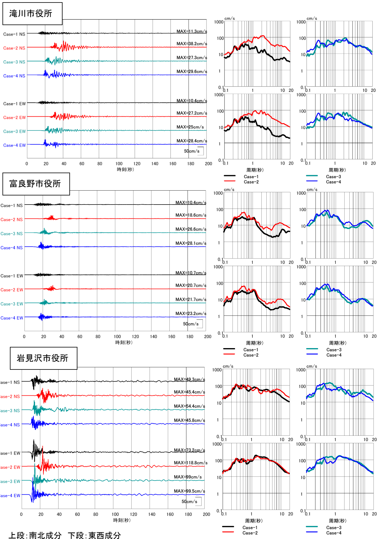
図 1 4 - 1 「詳細法工学的基盤」における計算波形と減衰 5 % 擬似速度応答スペクトル (滝川市役所・富良野市役所・岩見沢市役所)
