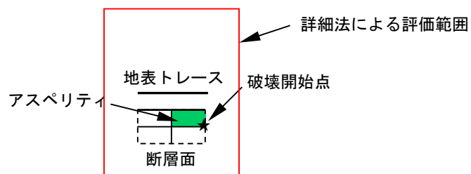
図 1 3 震源断層モデル (ケース 1 ~ 4)
