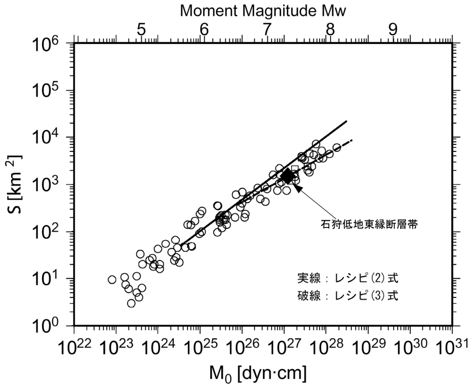
図 1 1 - 1 地震モーメント M_0 と断層面積 S との関係図
