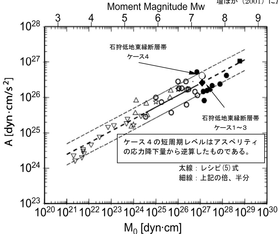
図 1 1 - 2 地震モーメント M_0 と短周期レベル A の関係図
