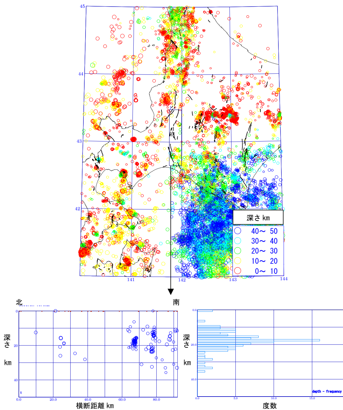
図 10-1 石狩低地東縁断層帯周辺の震央分布 (上図) および 震源分布の断面図 (下図左) 震源頻度分布図 (下図右)
