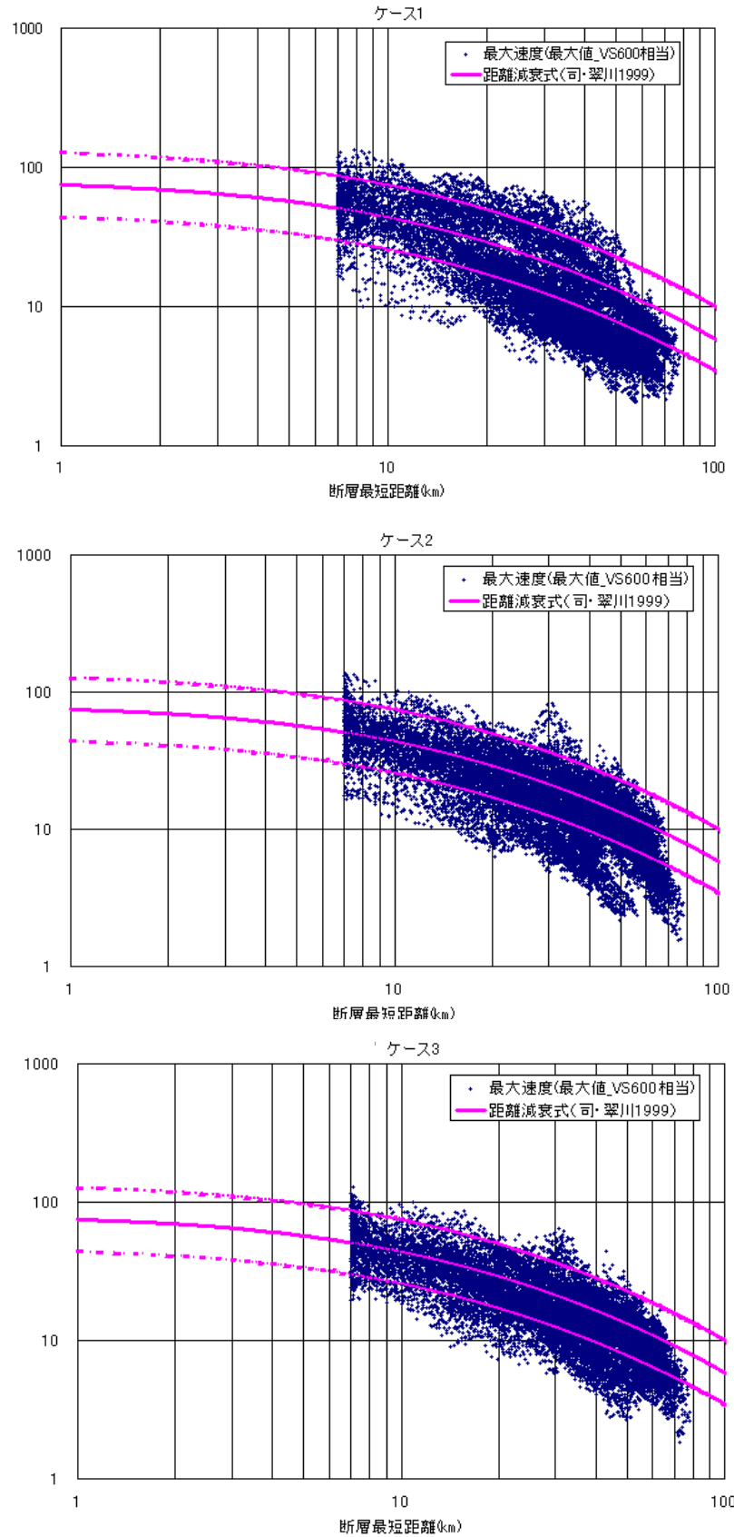
図6 「詳細法工学的基盤」(Vs=480m/s)における最大速度値をVs=600m/s相当に補正した値と司・翠川(1999)の距離減衰式との比較(ケース1~3)
