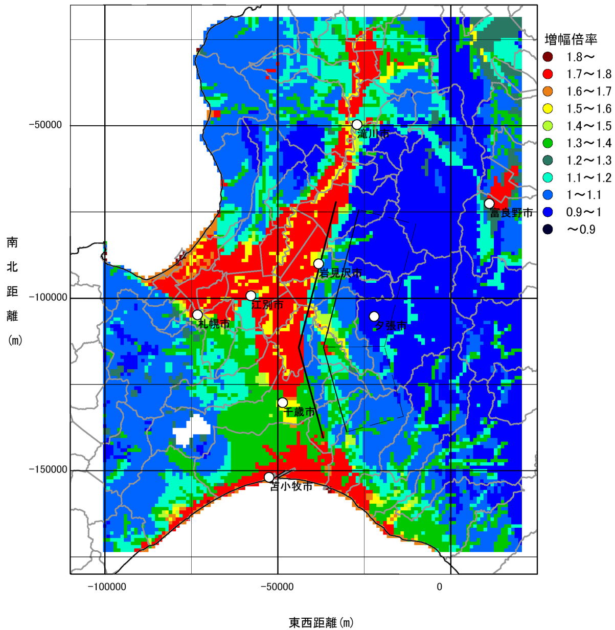
図4 「浅い地盤構造」(詳細法工学的基盤 ( V_s=480\text{m/s} 相当) から地表まで)での最大速度の増幅率の分布図
