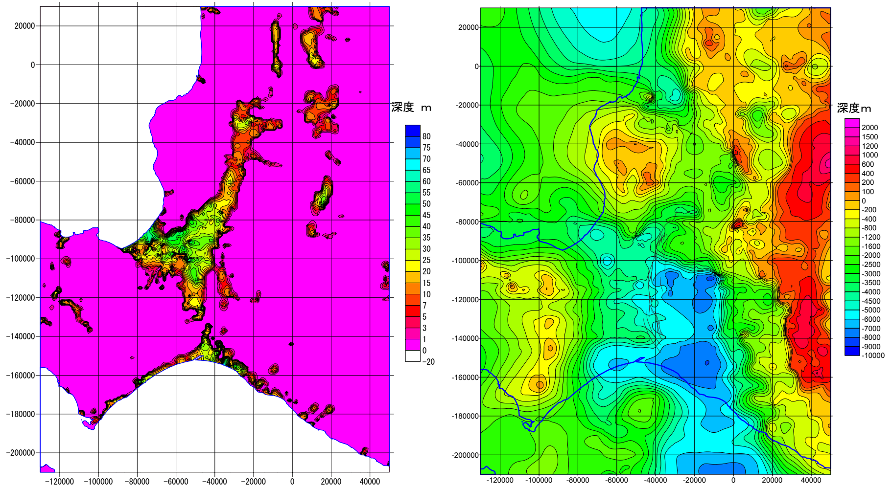
図3 詳細法工学的基盤等深線図（「浅い地盤構造」の基底面モデル： V_p=1.8\text{km/s} 上面，左図）と地震基盤等深線図（「深い地盤構造」の基底面モデル： V_p=5.7\text{km/s} 上面，右図）
