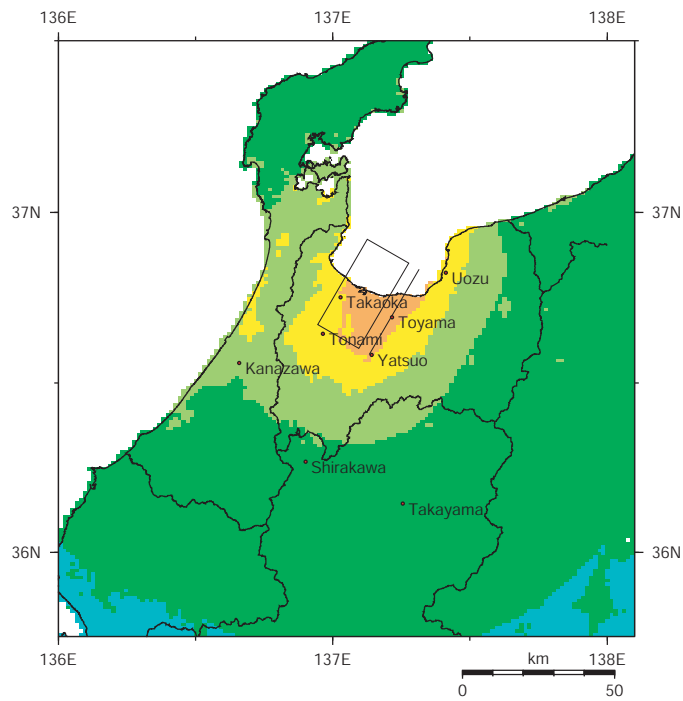
呉羽山断層帯
