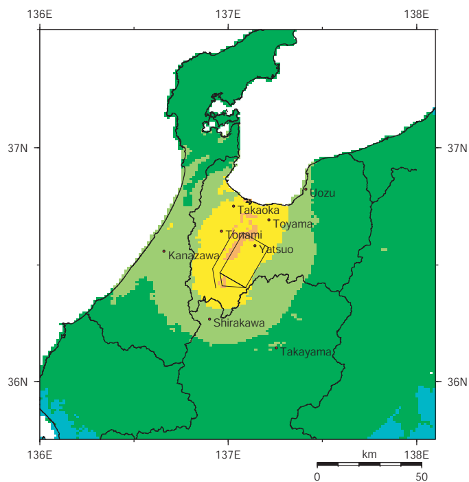
砺波平野断層帯東部
