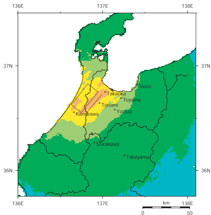
砺波平野断層帯西部
