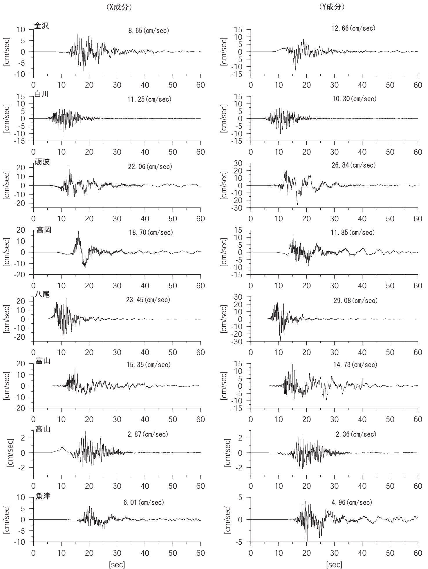
図 13-2 「詳細法工学的基盤」 ( V_s=450\text{m/s} ) における計算波形例 砺波平野断層帯東部 (アスペリティ2つ)
