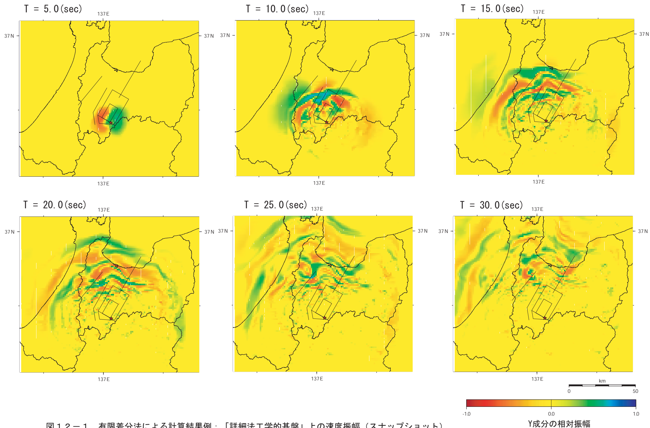
図 1 2 - 1 有限差分法による計算結果例：「詳細法工学的基盤」上の速度振幅（スナップショット） 砺波平野断層帯東部（アスペリティ 1 つ）
