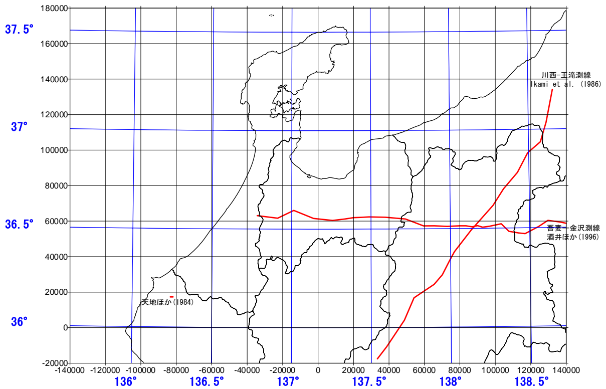
図 10-1 物理探査（屈折法地震探査）測線位置
