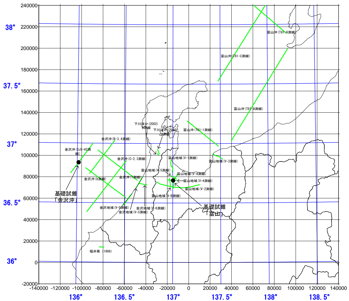
図 10-2 物理探査（反射法地震探査）測線位置
