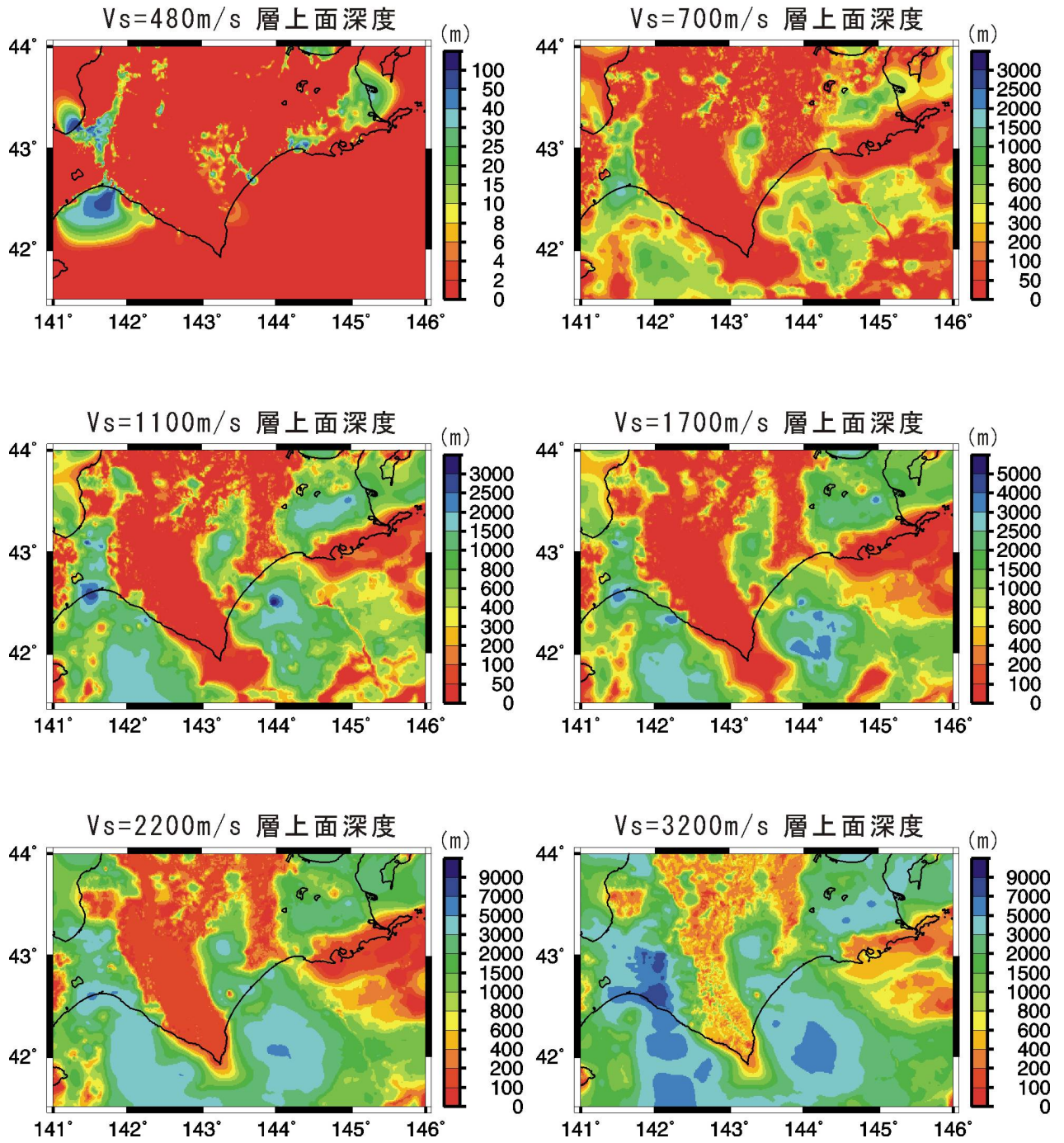
図3 「深い地盤構造」に用いた三次元地下構造モデル（各速度層上面の深さ分布）
