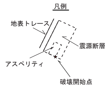
図18-2 「詳細法」による強震動予測結果：「詳細法工学的基盤」上の最大速度分布 武山断層帯：ケース3（左）、衣笠・北武断層帯：ケース4（右）
