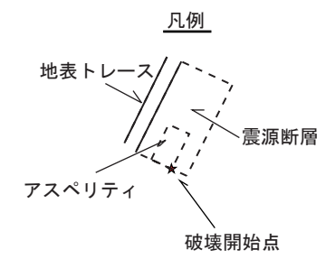
図18-1 「詳細法」による強震動予測結果：「詳細法工学的基盤」上の最大速度分布 武山断層帯：ケース1（左）、ケース2（右）
