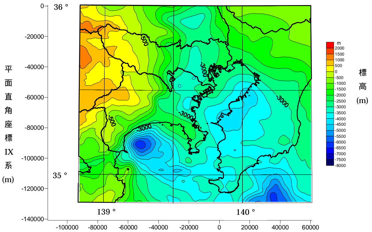
図14-1 速度層上面コンタ図 (上: V_s=3.2\text{km/s} 、下: V_s=2.8\text{km/s} )
