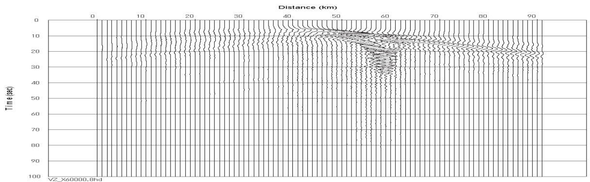
図 15-2 三次元地下構造モデル断面とその断面沿いの評価地点（地表）における時刻歴波形（図 12 の②とほぼ同じ位置の断面）
