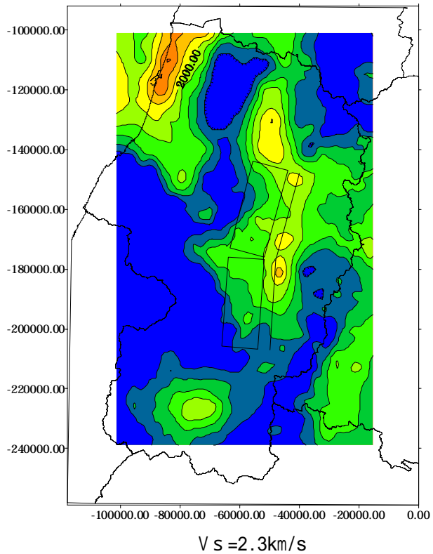
図 1 3 各速度層上面深さのコンタ図 (0m ~ 4000m を 400m ピッチで表現)
