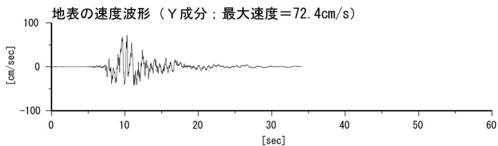
図 2 4 - 1 地表における時刻歴波形の計算例（ケース 1 a）
