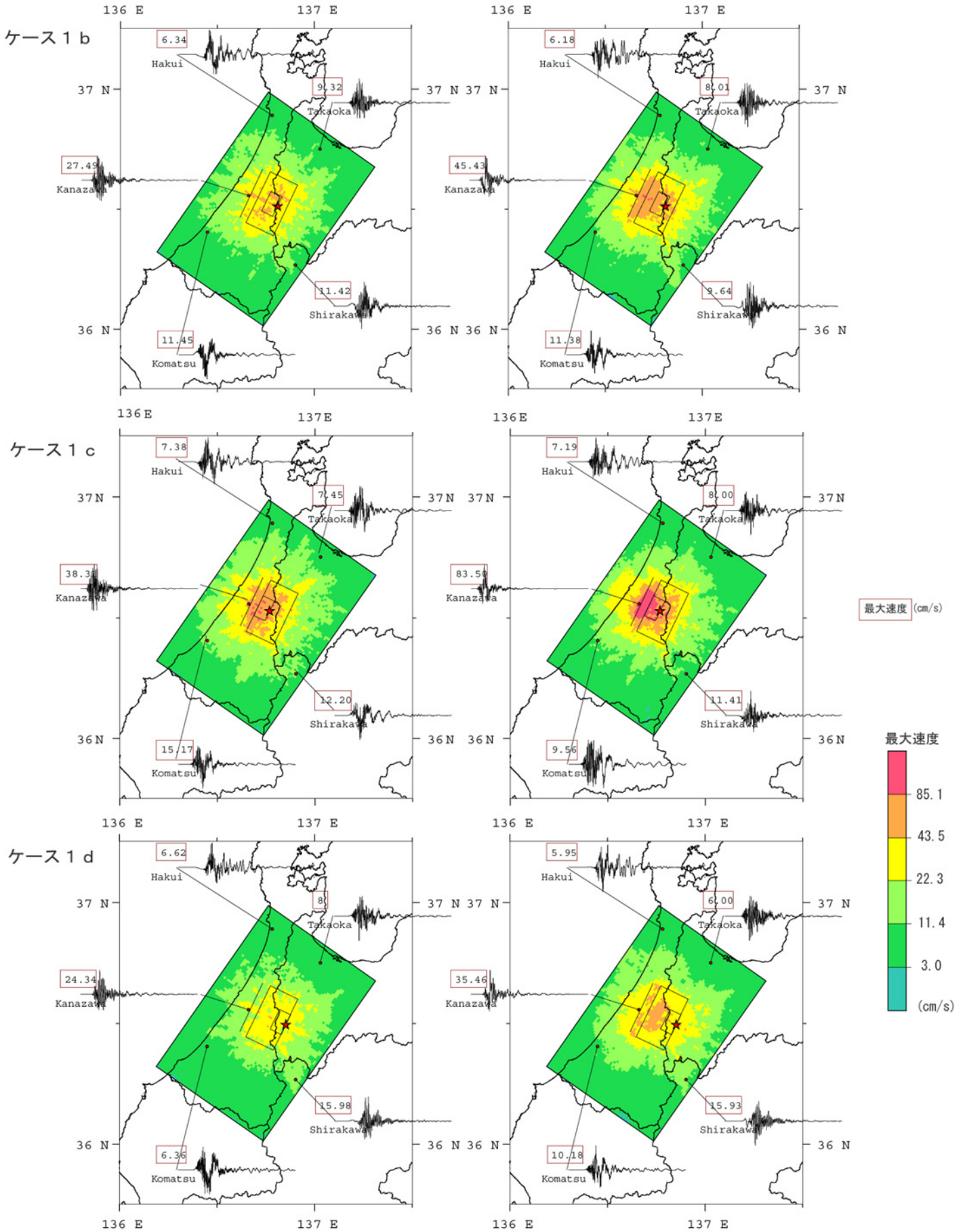
図16-2 詳細法による強震動予測結果 「詳細法工学的基盤」上の最大速度分布
