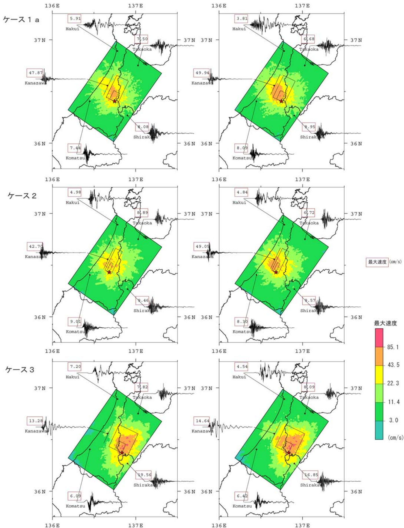
図16-1 詳細法による強震動予測結果 「詳細法工学的基盤」上の最大速度分布
