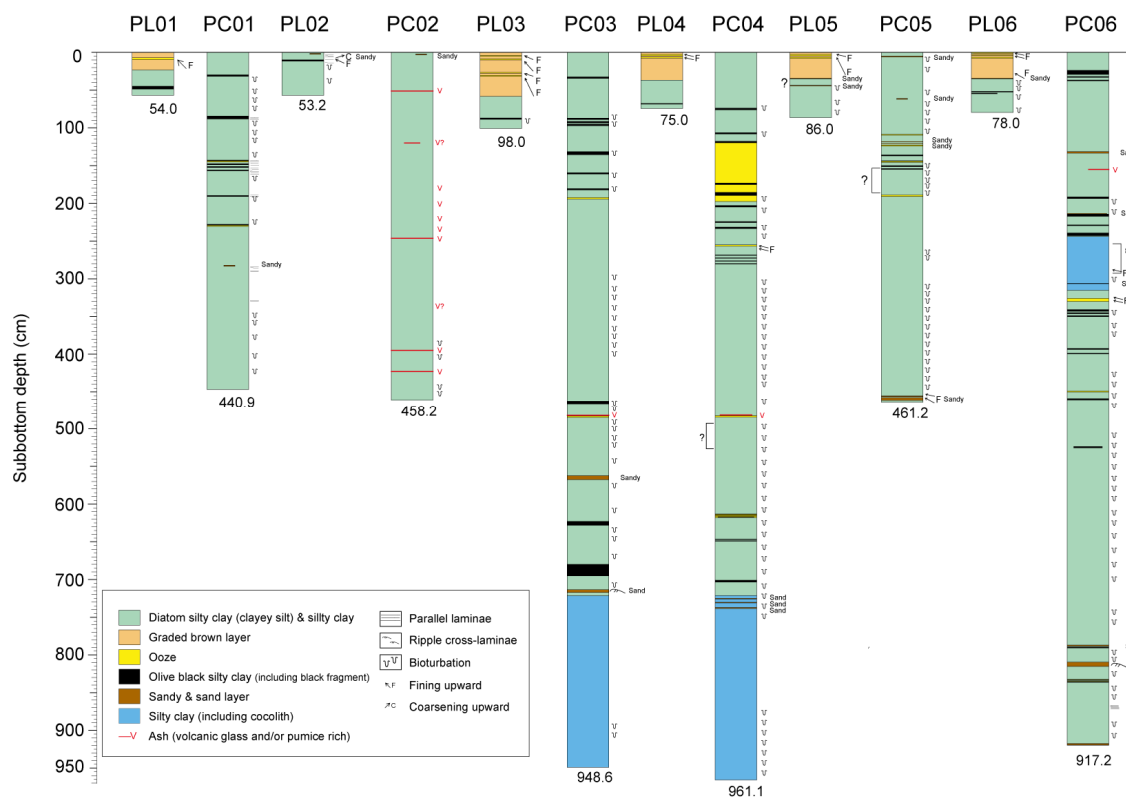
図2 MR12-E01によって採取されたコアの岩相図の概要。PCはピストンコアラー本体を示す。PLはパイロットコアラーで表層を乱すことなく試料採取した。
