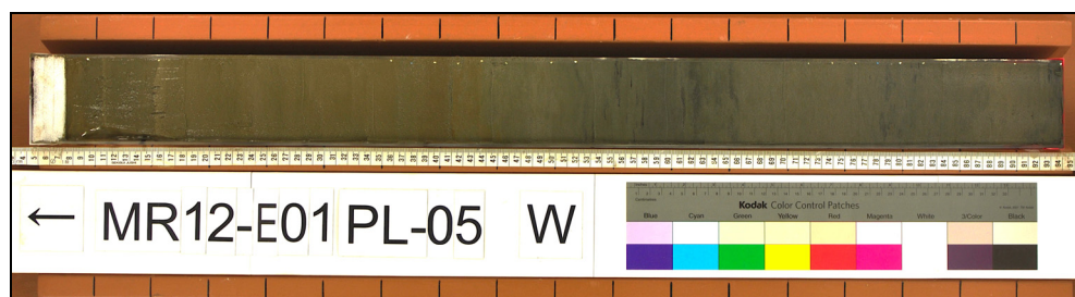
図3 “地形的高まり”より採取されたコアのごく表層部のコアの写真 左がコアの最上部、(ごく表層 90cm) には乱れた様子はない。
