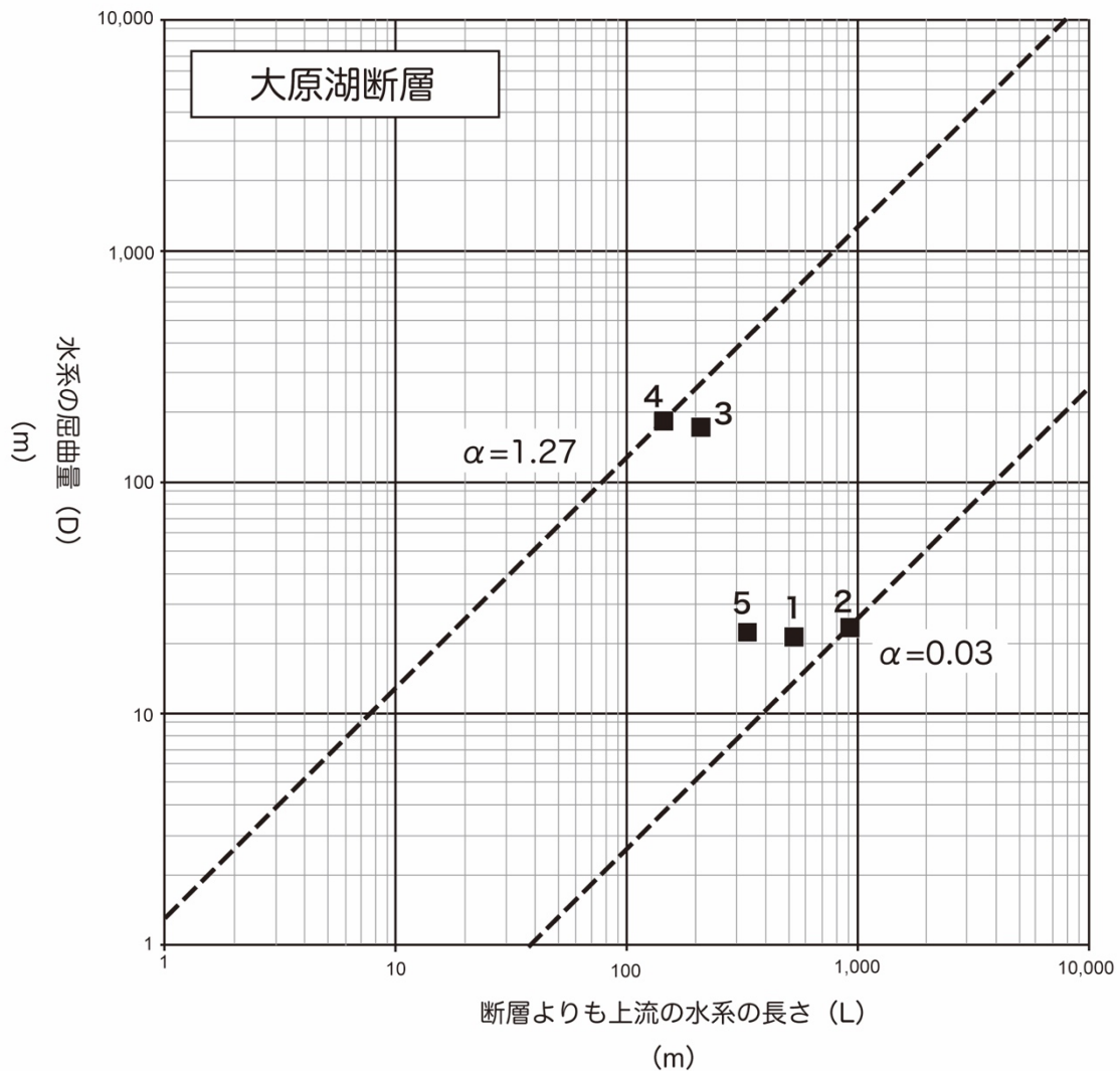
図3 大原湖断層における水系の屈曲量 (D) と上流の長さ (L) との関係 数字は地形解析を行なった地点の番号を示す。各地点の位置は図2に示す。
