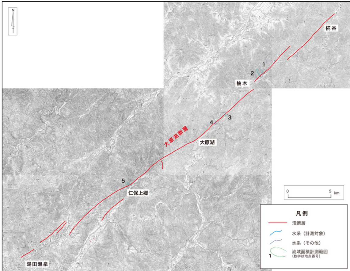
図2 大原湖断層を横切る水系と地形解析を行なった地点 活断層の位置は地震調査研究推進本部地震調査委員会（2016a）にしたがった。
