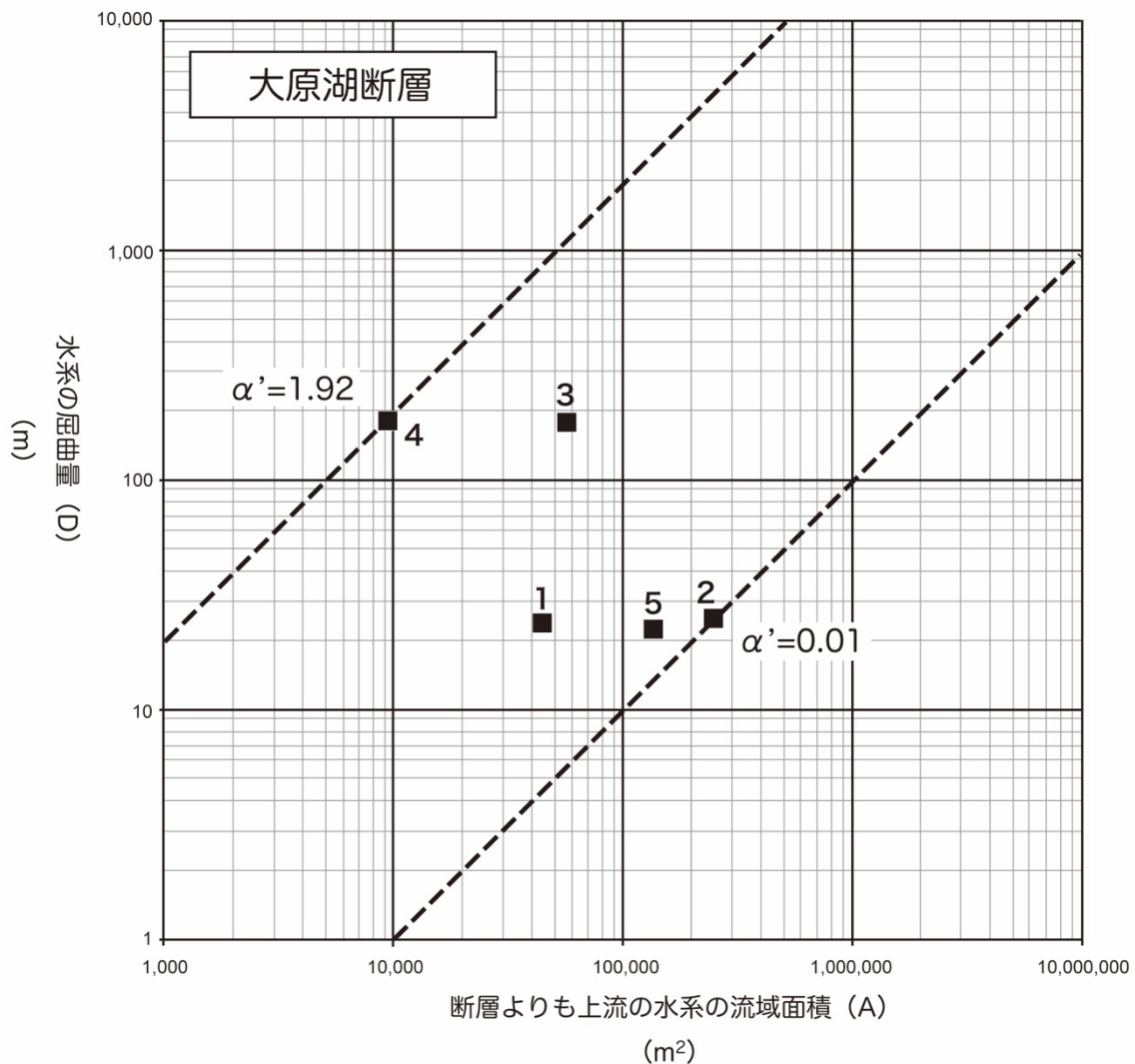
図4 大原湖断層における水系の屈曲量 (D) と上流の流域面積 (A) との関係 数字は地形解析を行なった地点の番号を示す。各地点の位置は図2に示す。
