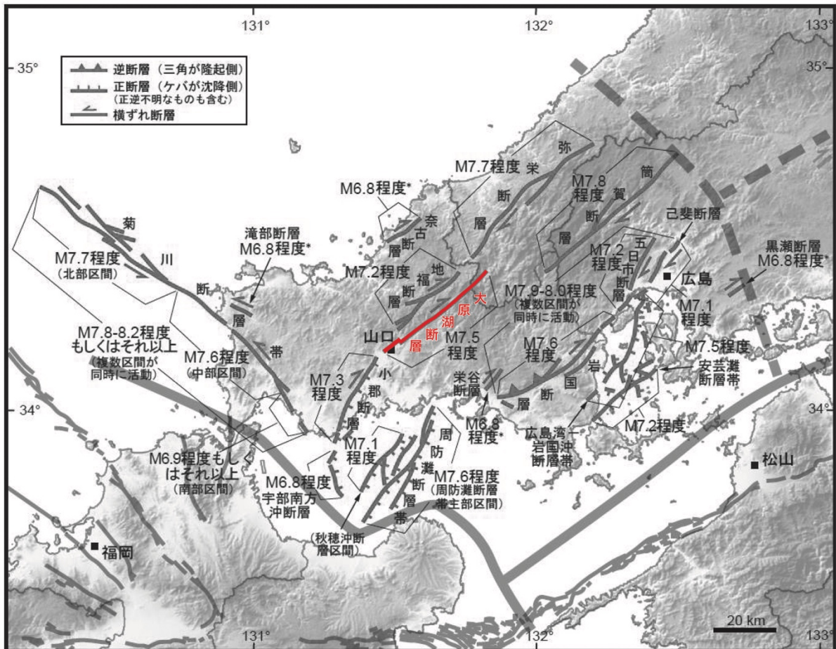
図 1 大原湖断層の位置 (地震調査研究推進本部地震調査委員会(2016a)を改変) 大原湖断層の位置を赤線で示した。
